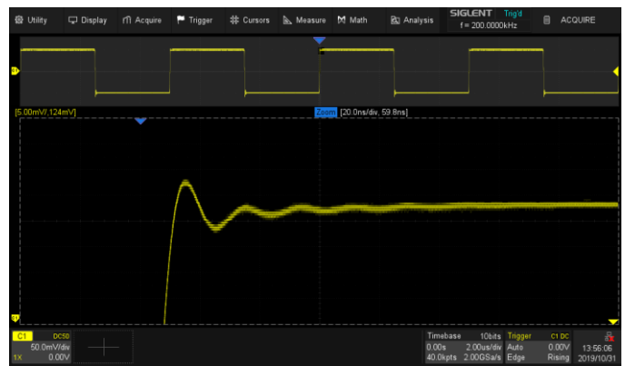
10-bit 模式
